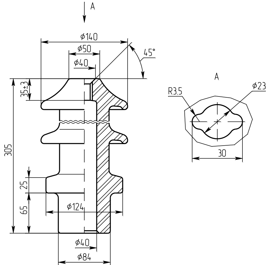
ИПТ-10/630 Б 01 чертеж ИВЕЮ.757524.048-01 креслення
